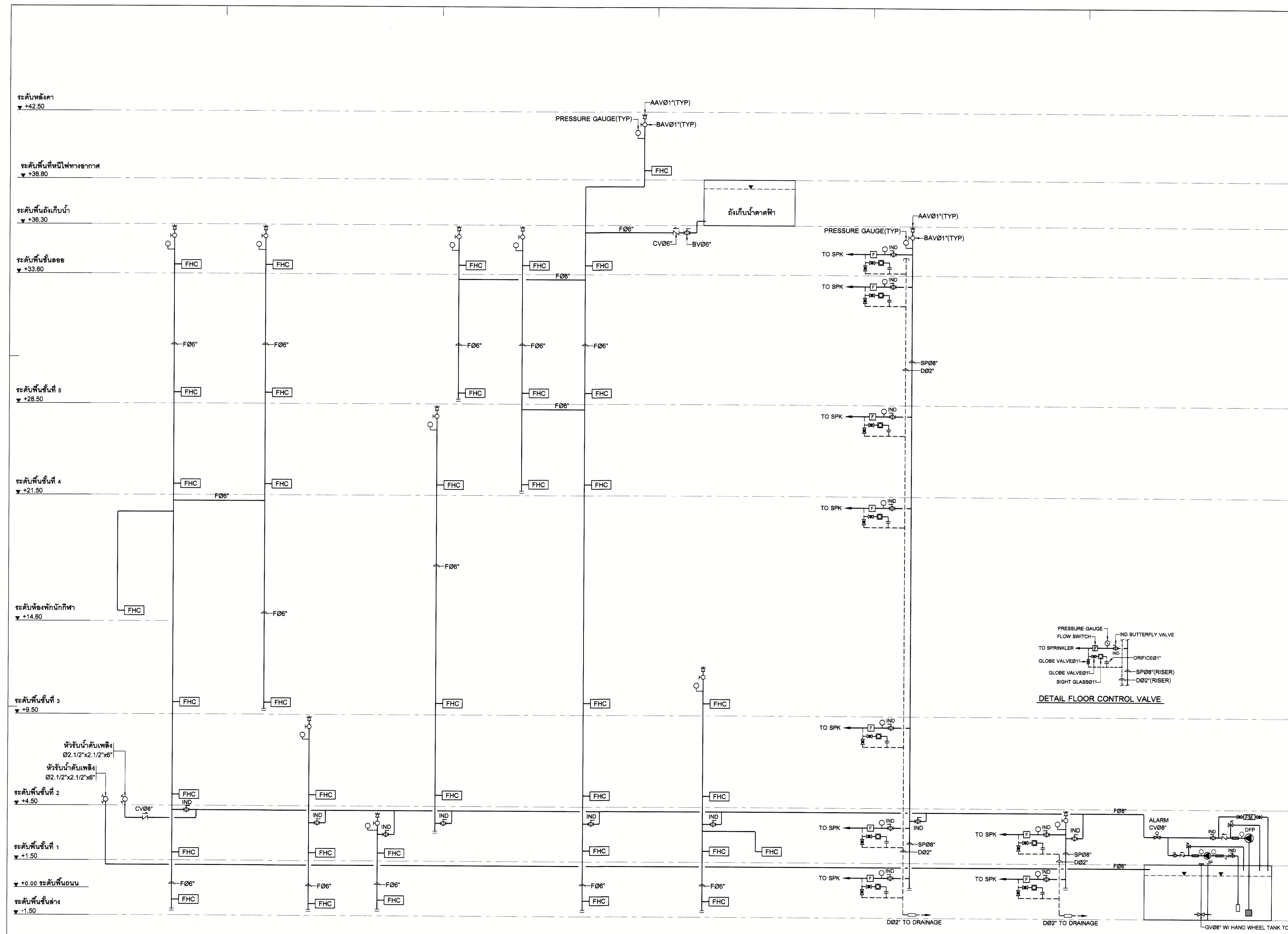
ไดอะแกรมระบบป้องกันอัคคีภัย
