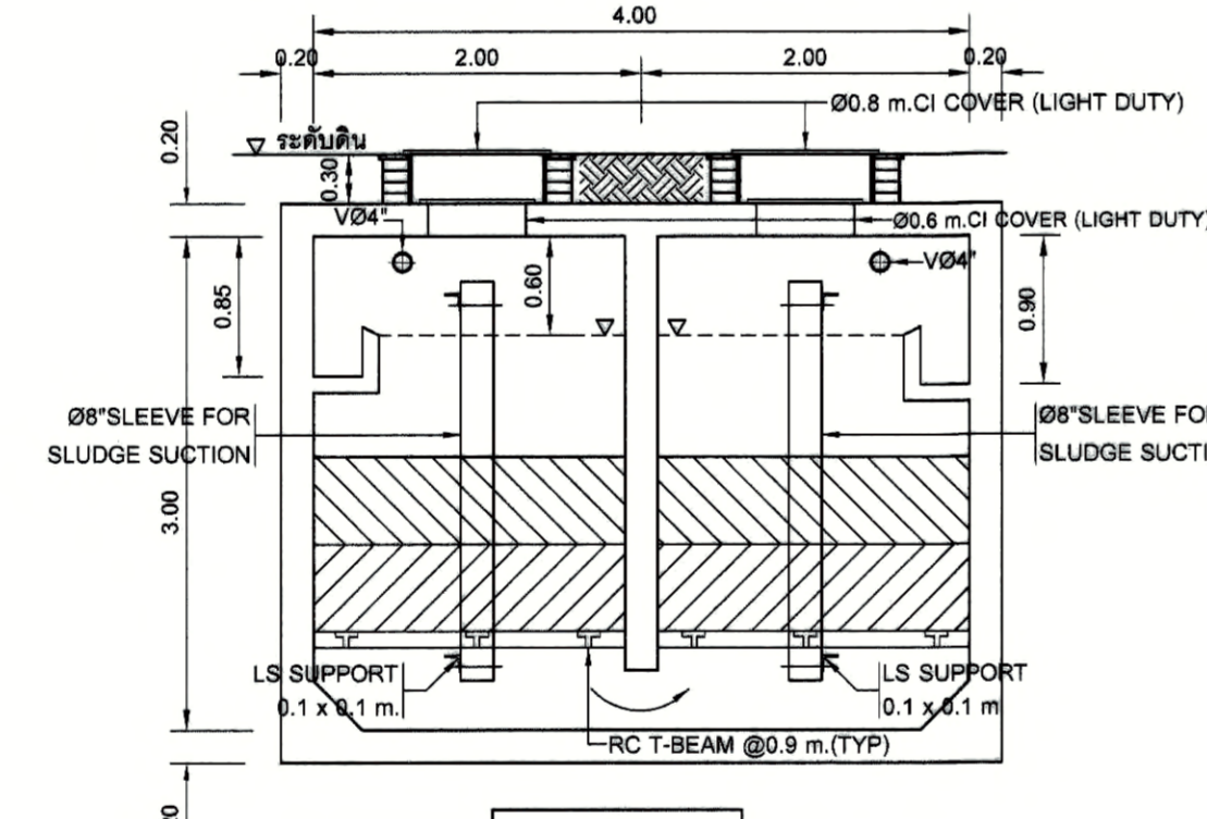
รูปตัด 4-4 มาตราส่วน 1:50
