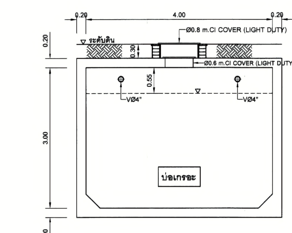
รูปตัด 3-3 มาตราส่วน 1:50
