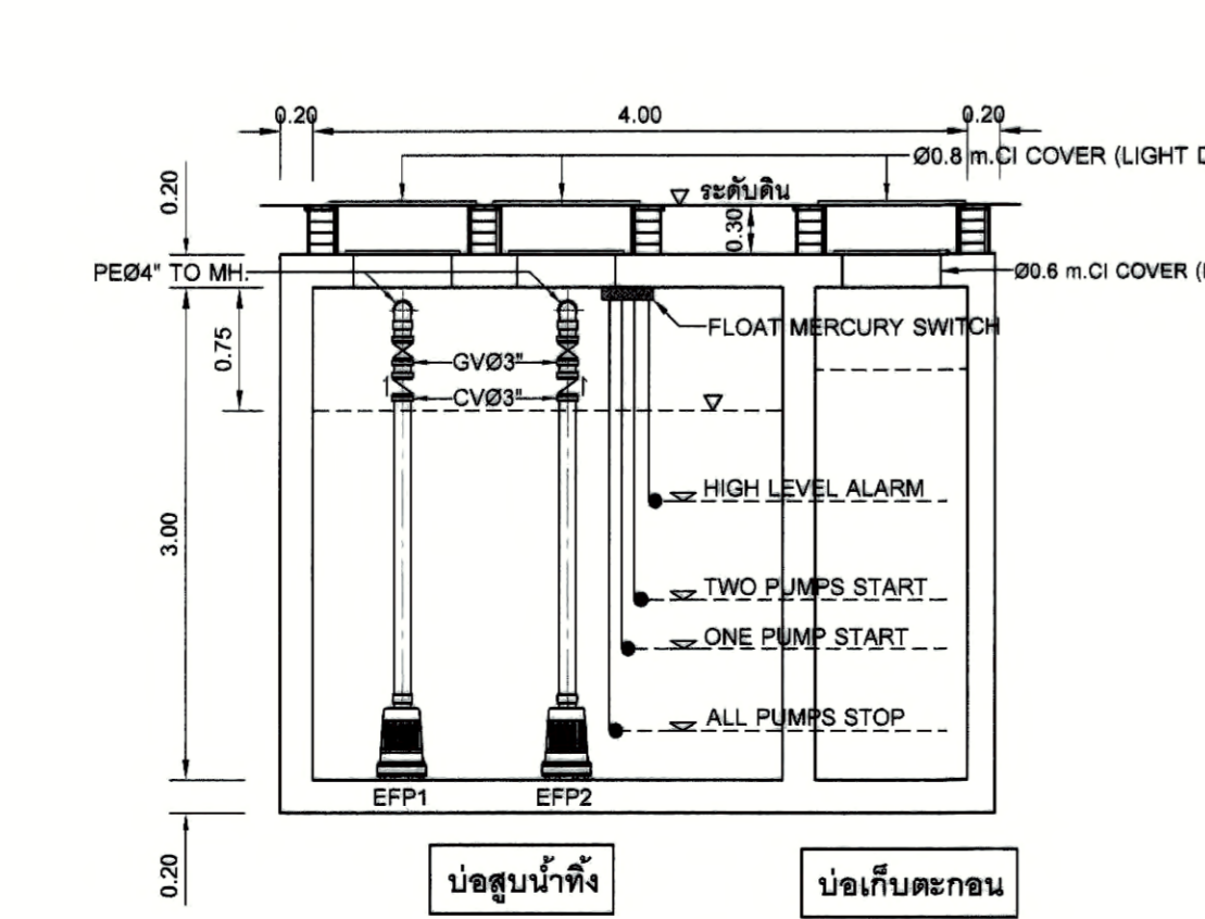
รูปตัด 7-7 มาตราส่วน 1:50
