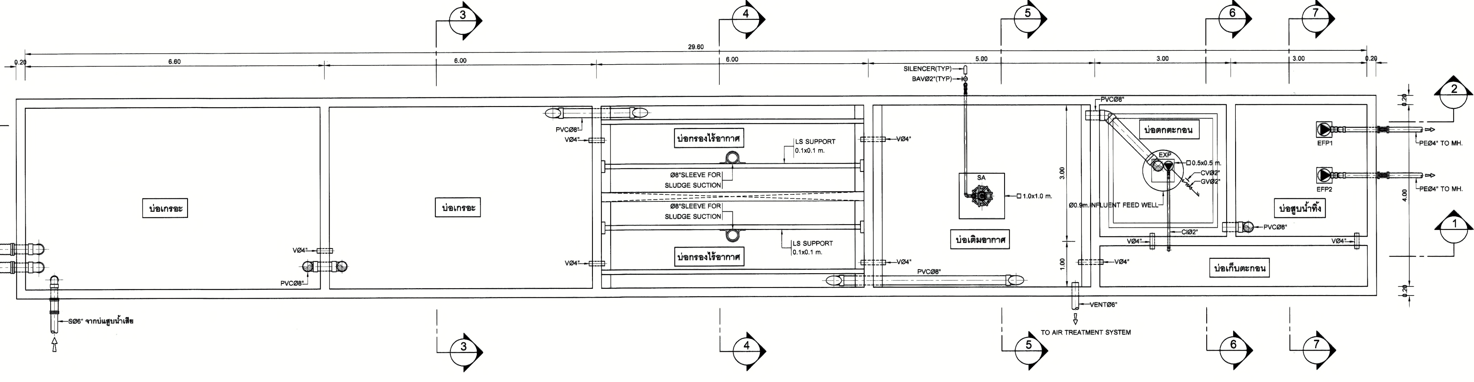
แปลนบ่อบำบัดน้ำเสีย มาตราส่วน 1:50
