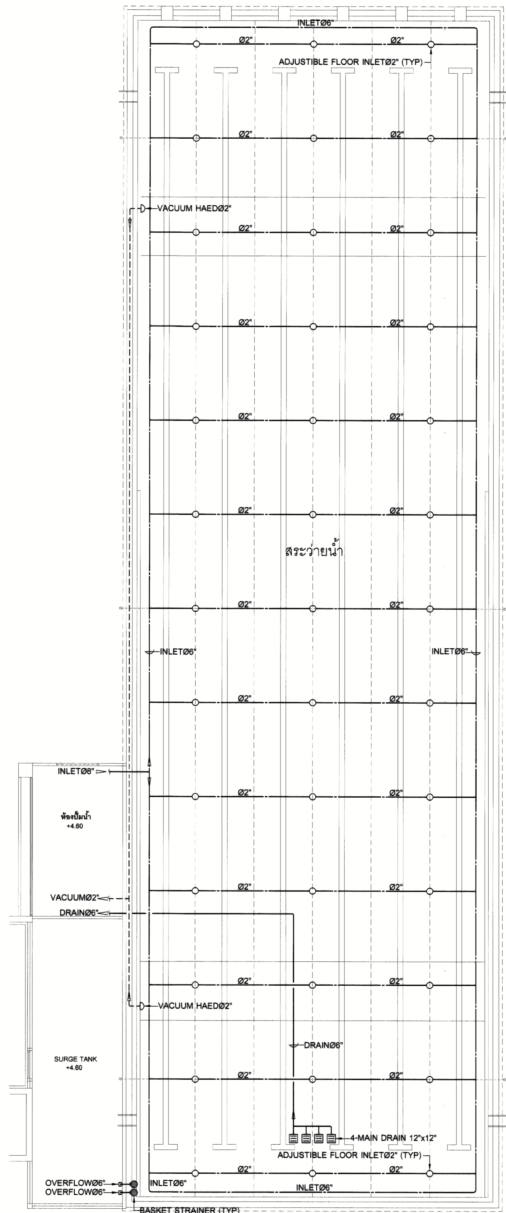
ฝัังสระว่ายน้ำ มาตราส่วน 1:100
