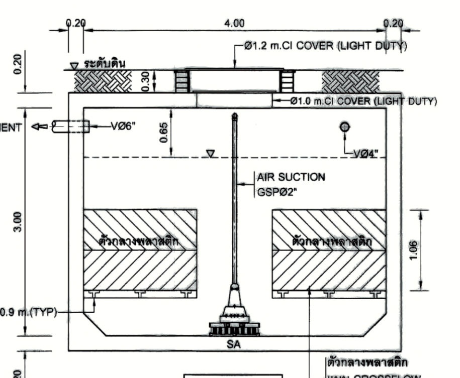
รูปตัด 5-5 มาตราส่วน 1:50
